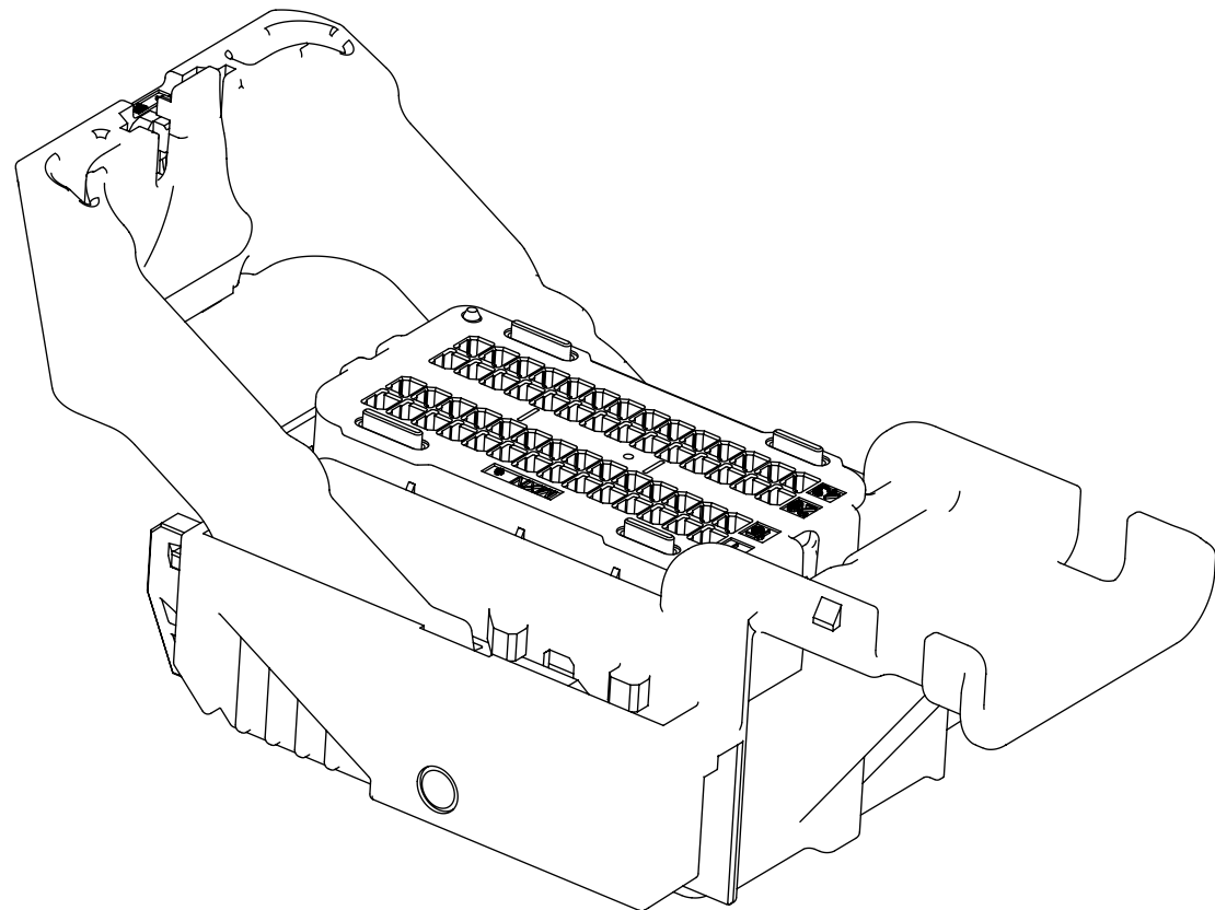
56 CKT SCALE 1.5:1
