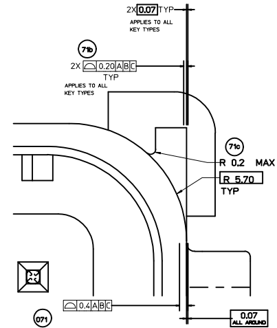
DETAIL Y
