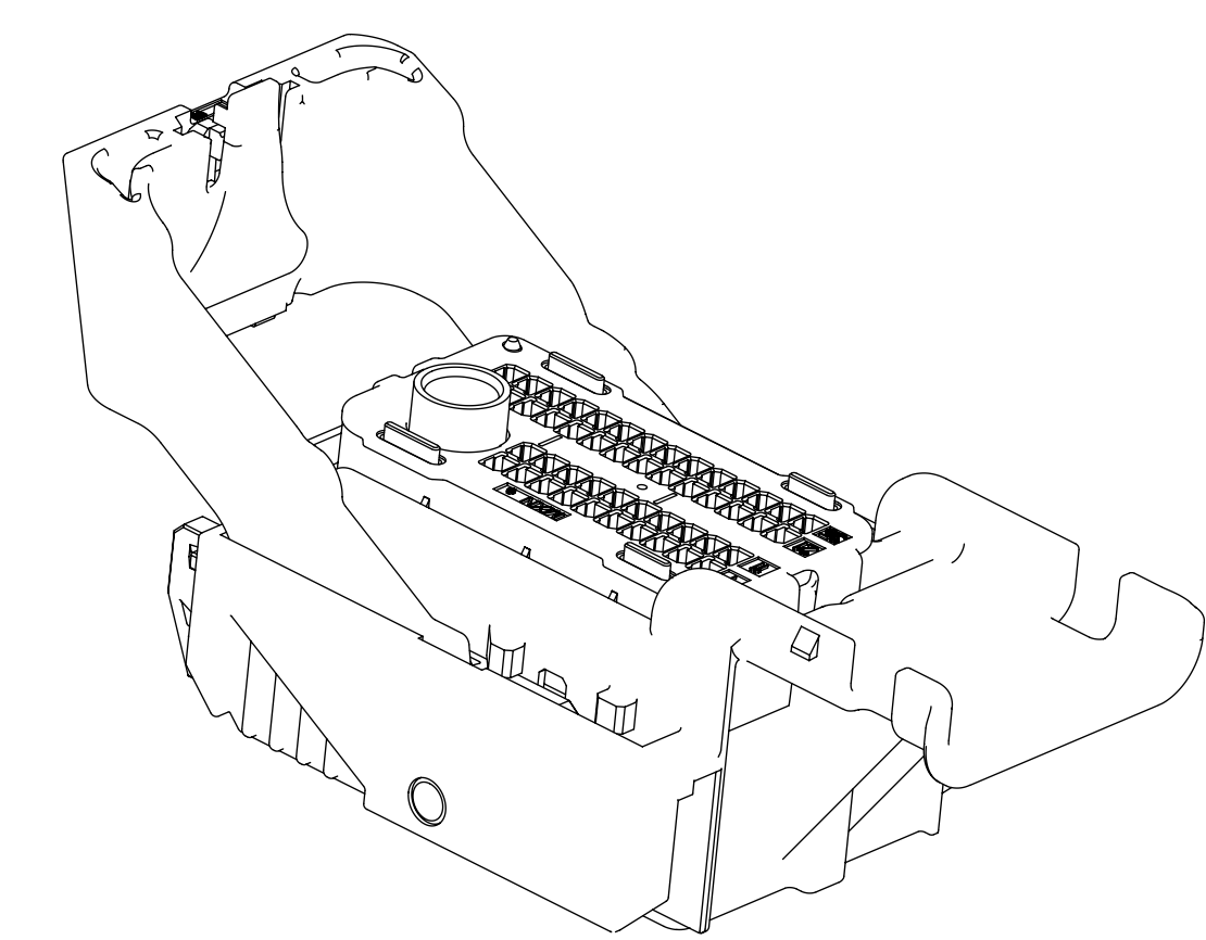
49 CKT SCALE 1.5:1
