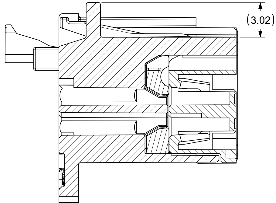
SECTION D-D
